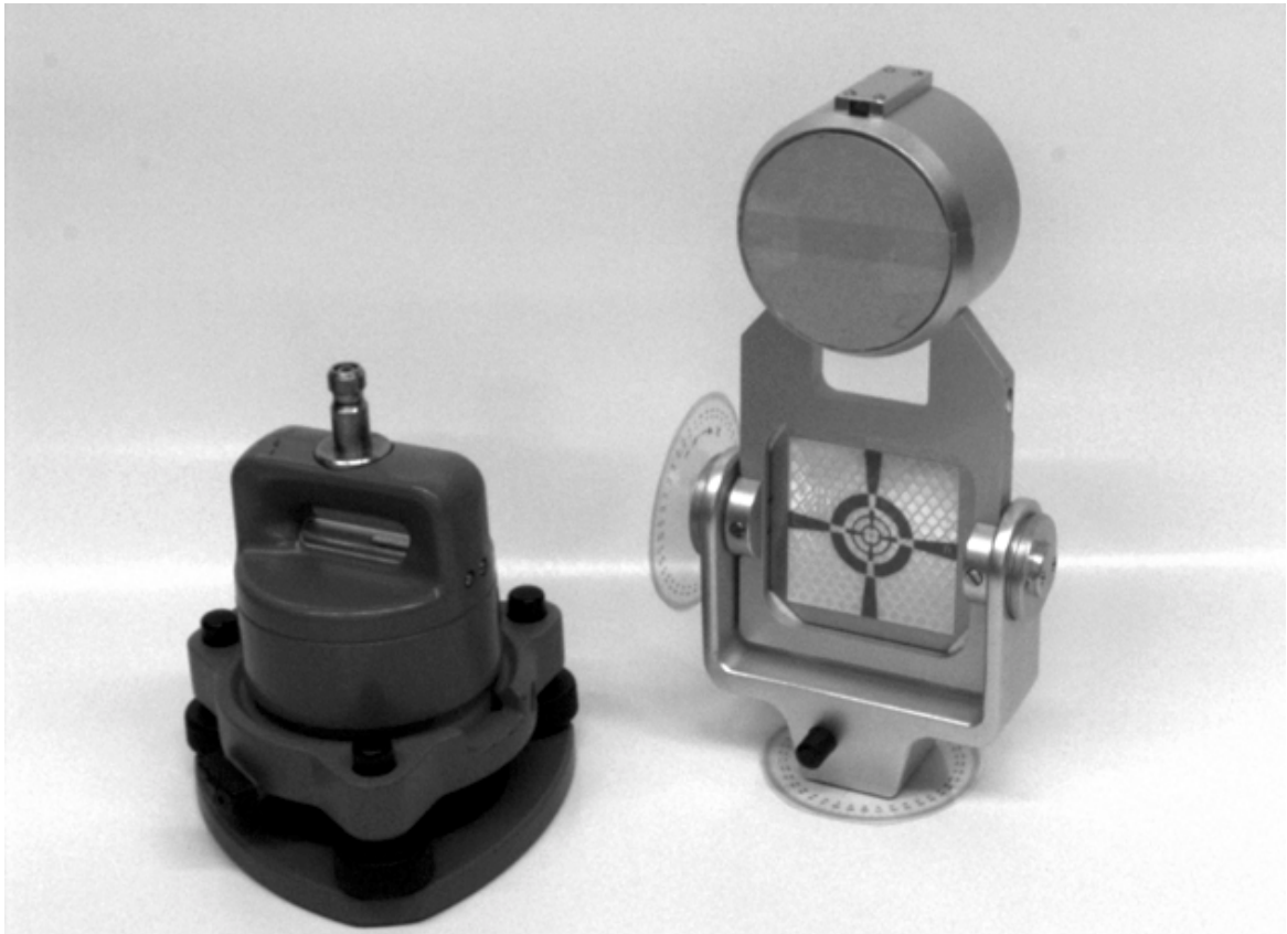
Abb.: Um zwei Achsen drehbarer Träger mit GOECKE Reflexionszielmarke
